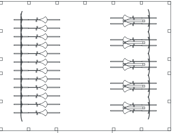
Ruimte voor 12 fietsen met een bevestigingsbeugel en 10 fietsen met een leunbeugel.
